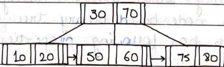
B+ tree
